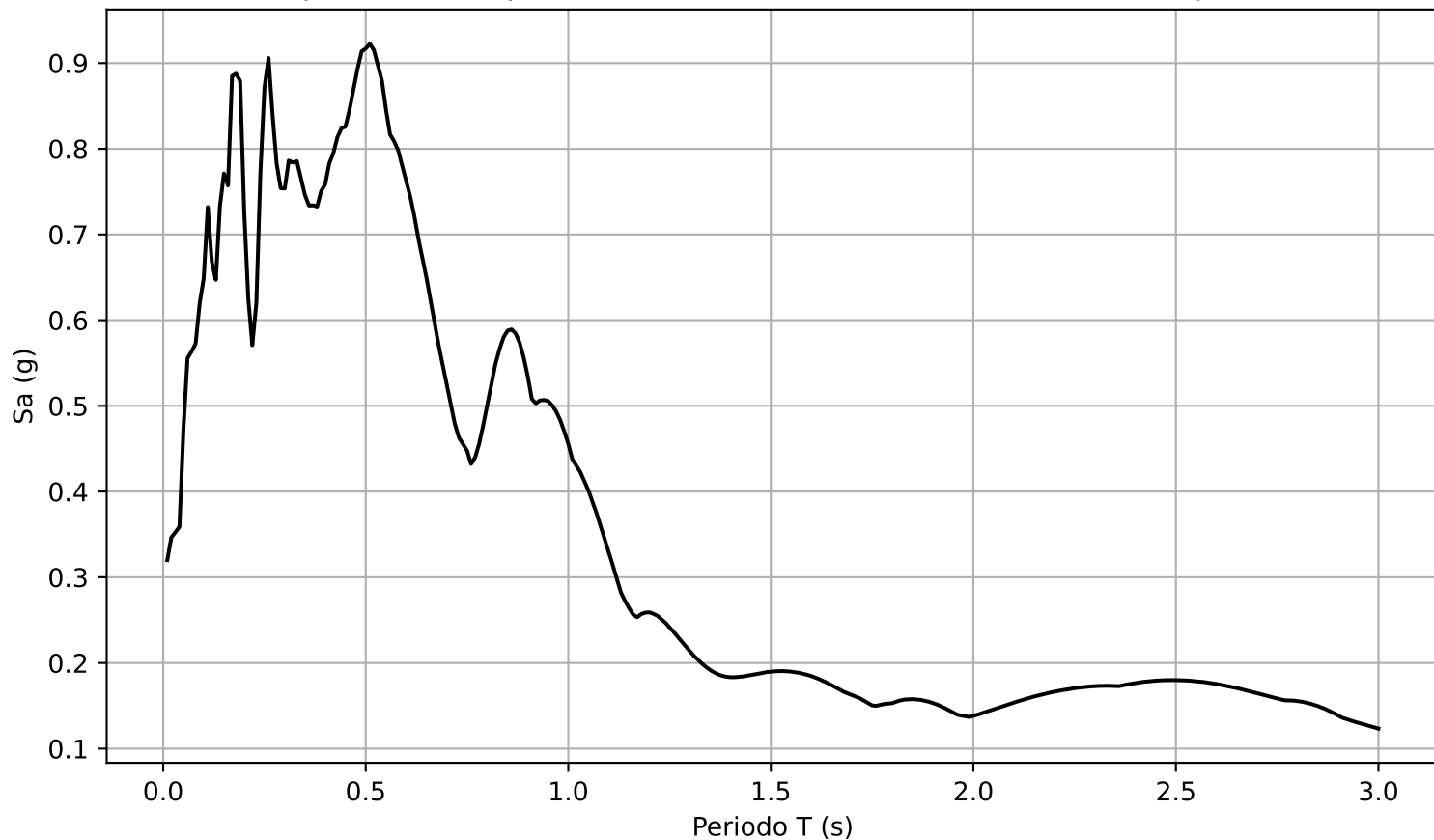
Espectro de respuesta de aceleraciones - El Centro (1940), \zeta=5\%
